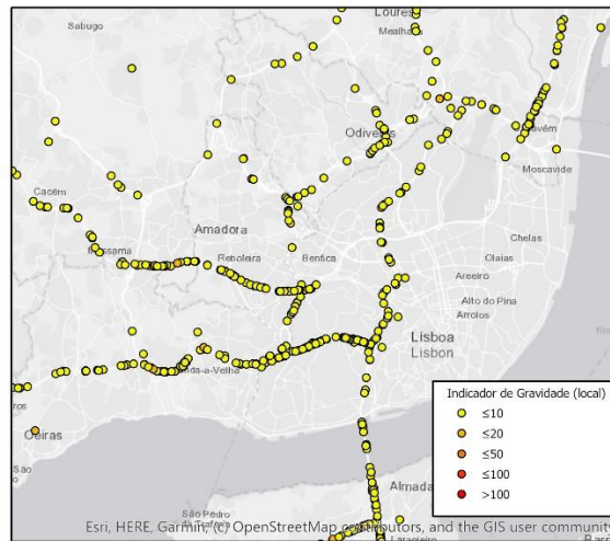
Figura 80: Indicador de Gravidade (local) dos acidentes na Rede Nacional de Autoestradas (2019)
